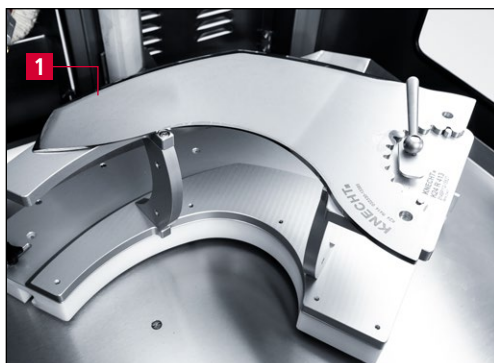
Rys. 7-5 Mocowanie noża
