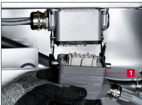
Bild 9-5 Verbindungsstecker Gleitblech lösen
