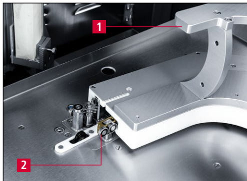
Bild 7-56 SP 112 Kopierschleifplatte auf Führungswagen schieben
