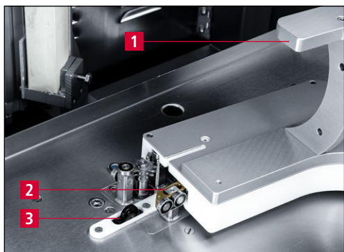
Bild 7-28 SP 112 Kopierschleifplatte montieren
