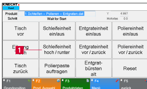
Bild 7-9 Hauptbildschirm
