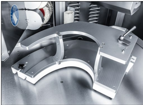
Bild 3-5 SP 112 Kopierschleifplatte
