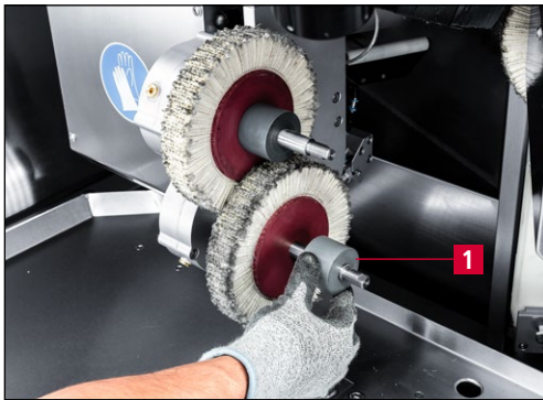
Bild 7-75 Zwischenflansch abnehmen
