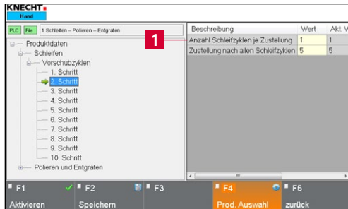
Bild 8-27 Produktdaten „Schleifen – Vorschubzyklen – 2. Schritt“
