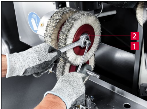
Bild 7-72 Gewindemutter lösen
