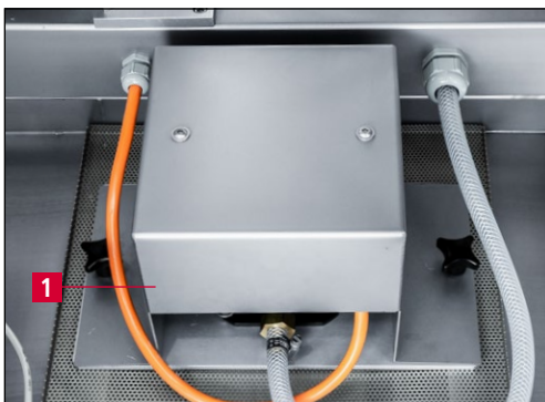
Bild 3-6 Kühlmittelpumpe
