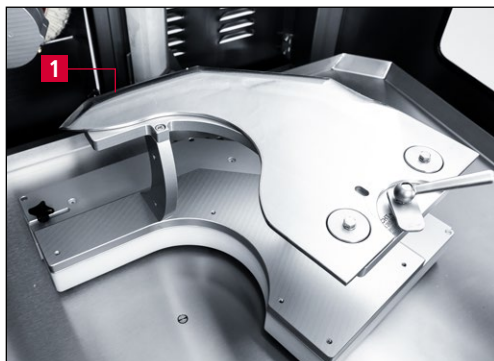
Bild 7-31 Messer aufspannen
