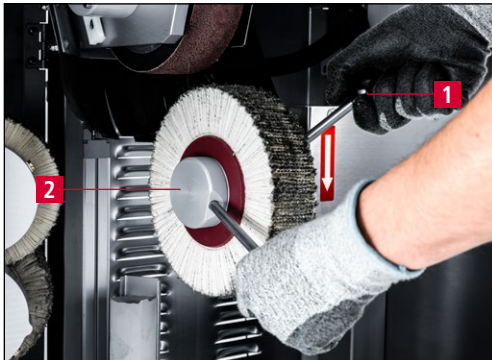
Bild 7-65 Polierbürste wechseln
