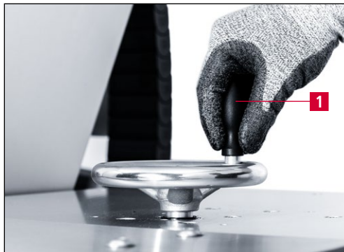
Bild 7-20 Höheneinstellung Poliereinheit
