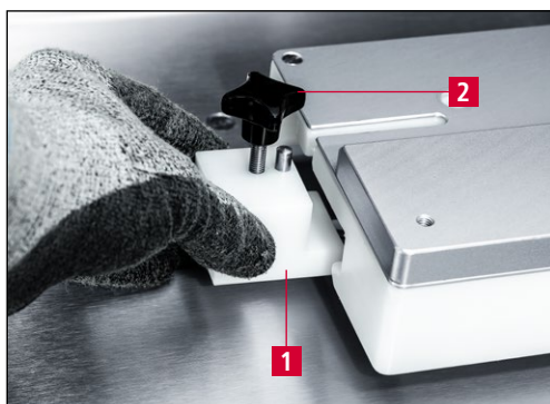
Bild 7-58 Endschalternocken anbringen
