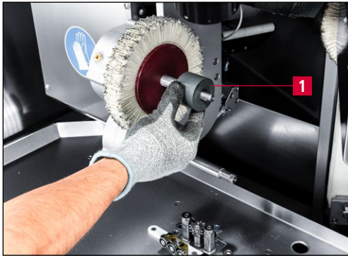
Bild 7-77 Zwischenflansch abnehmen
