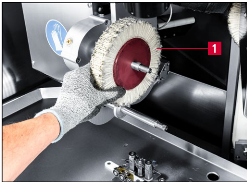
Bild 7-78 Obere Entgratbürste abnehmen
